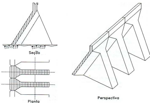
Figura 01 - Barragem de contrafortes. Fonte: Oliveira & Brito (1998)
